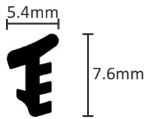
P41 Wedge
