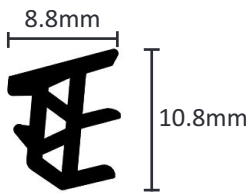
P115 Wedge
