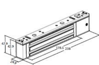
Z4 Electromagnetic Lock
